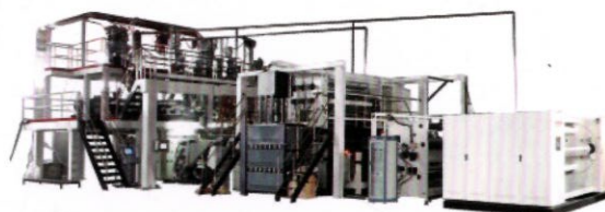
■ PE 透气膜生产线 PE Breathable Film Line
